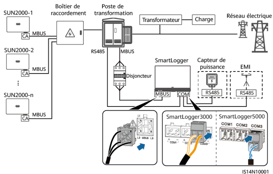
Figure 5-33 Communication MBUS (scénarios à l'échelle industrielle)
