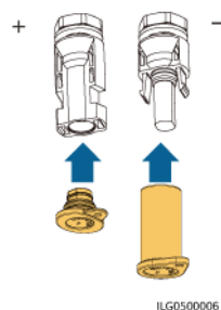
Figure 5-25 Bouchons d'étanchéité
