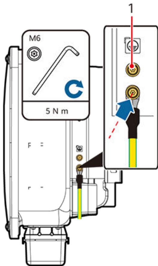
Figure 5-3 Raccordement du câble PE
