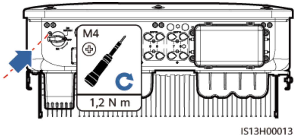
Figure 4-14 Installation de la vis de verrouillage du commutateur CC
