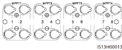
Figure 5-14 Bornes d'entrée CC
