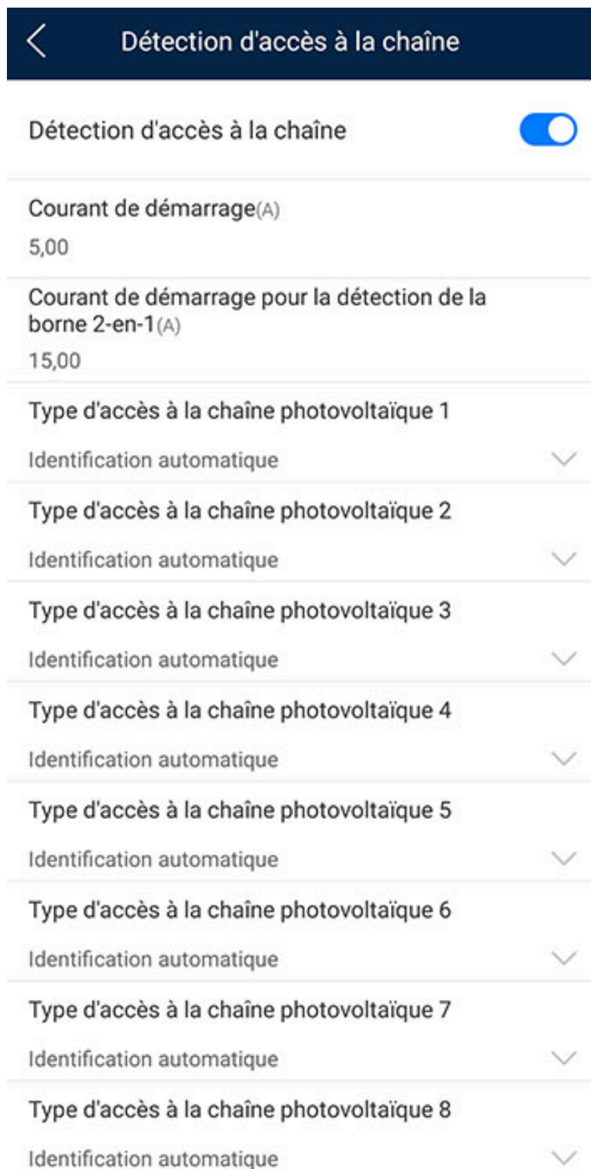
Figure J-1 Détection d'accès à la branche PV
