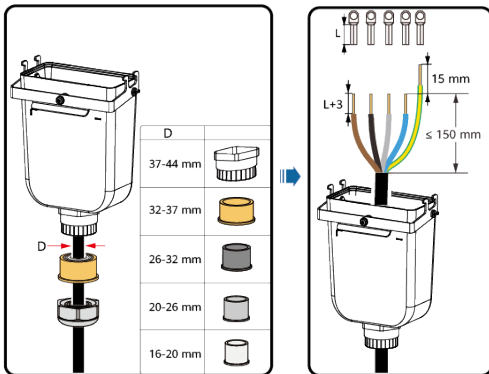
Figure 5-8 Dénuder un câble d'alimentation CA (en prenant comme exemple un câble à cinq conducteurs)
