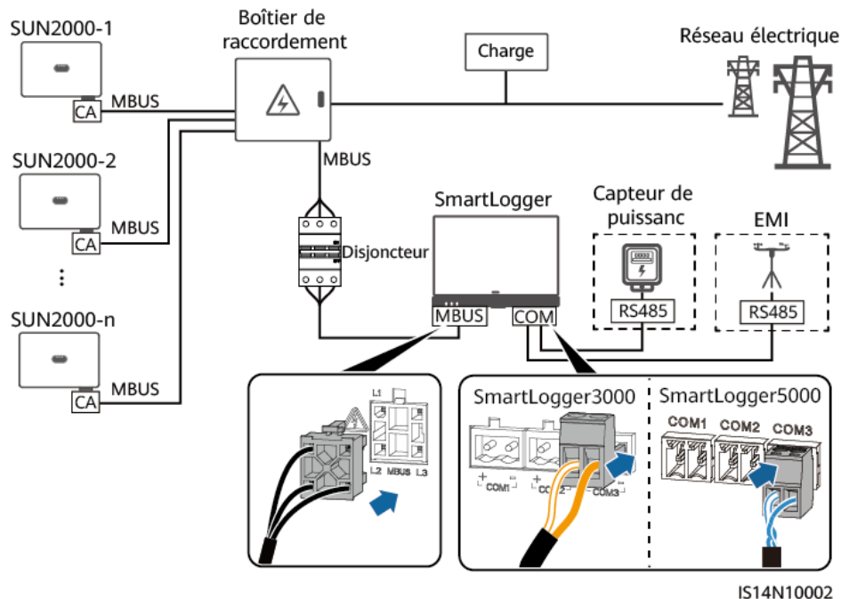
Figure 5-34 Communication MBUS (scénario C&I en Chine)
