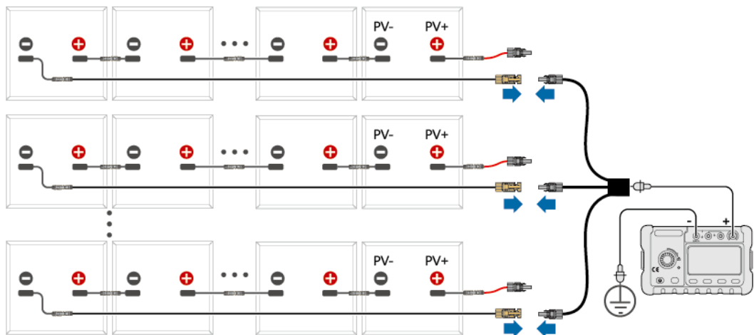
Figure 5-20 Mesure de la résistance d'isolation du PV– pour toutes les chaînes PV
