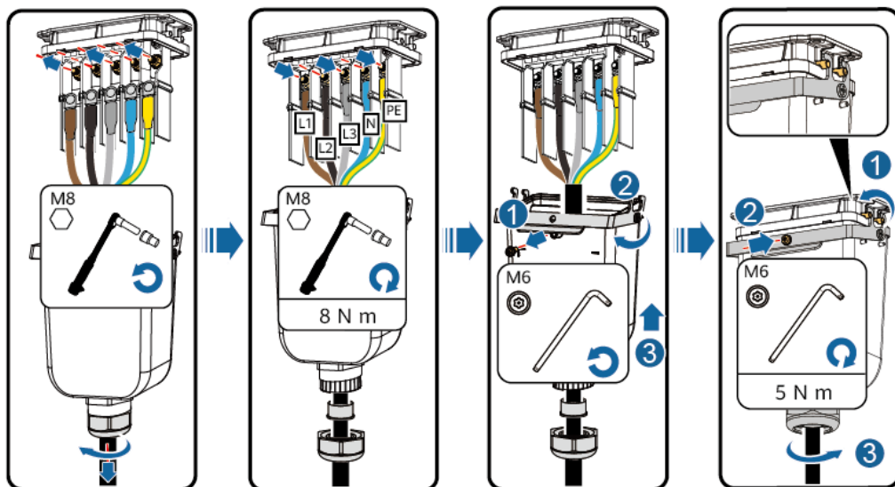
Figure 5-9 Câble à cinq conducteurs (L1, L2, L3, N et PE)
