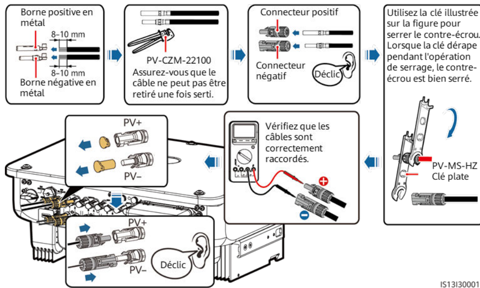
Figure 5-24 Connexion des câbles d'alimentation CC
