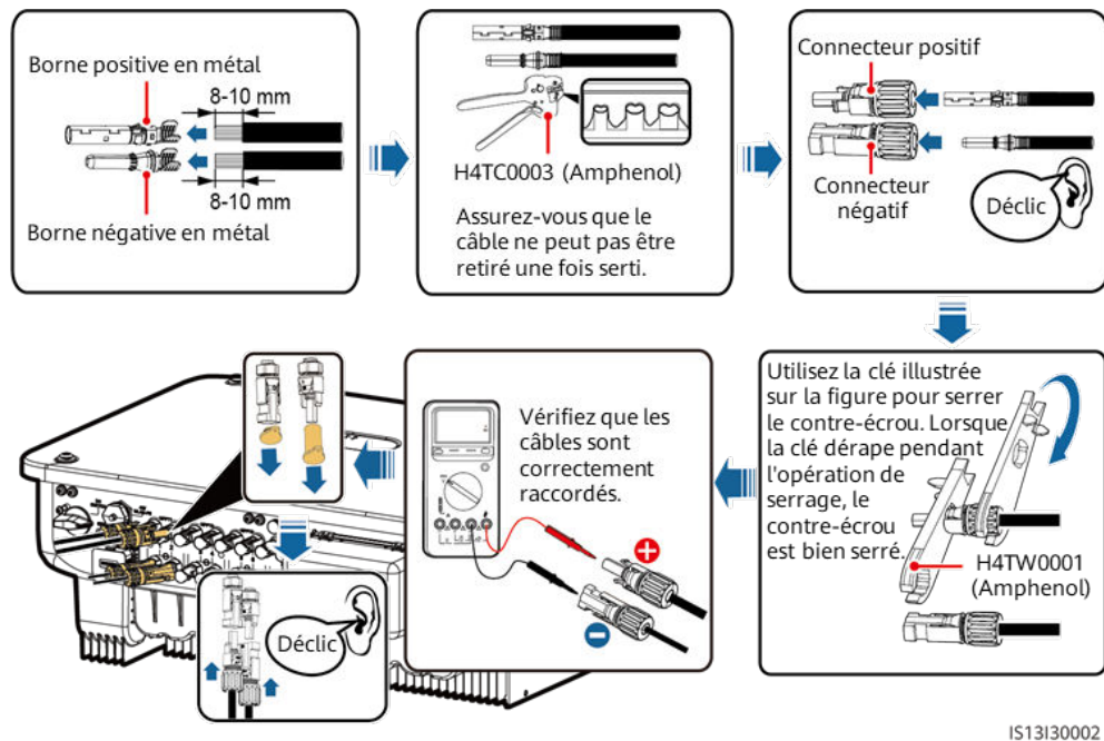
Figure 5-22 Connexion des câbles d'alimentation CC
