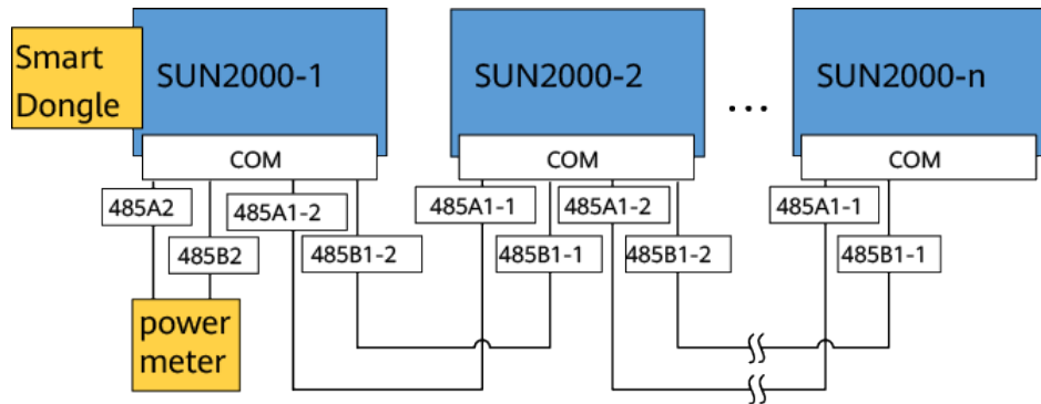
Figure 5-31 Mise en réseau du Smart Dongle
