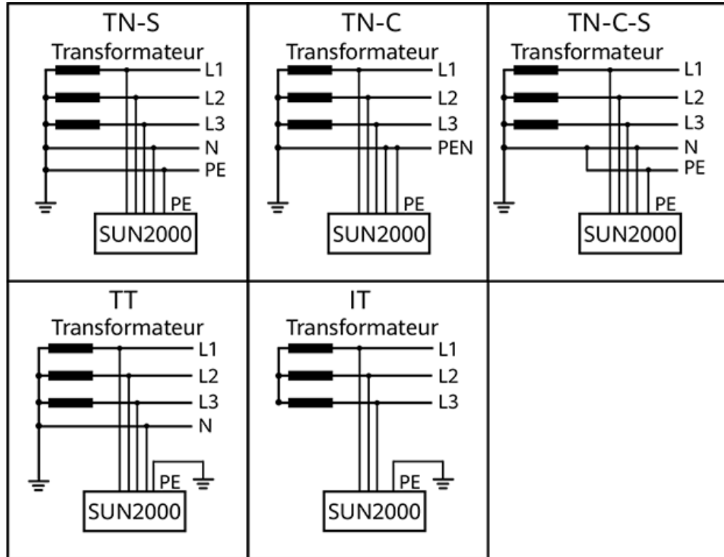
Figure 2-3 Systemes de mise à la terre
