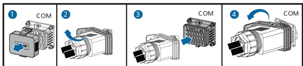
Figure 5-36 Fixation du connecteur du câble de signal
