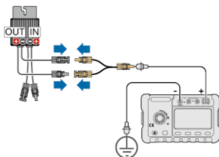
Figure 5-18 Mesure de la résistance d'isolation de l'optimiseur
