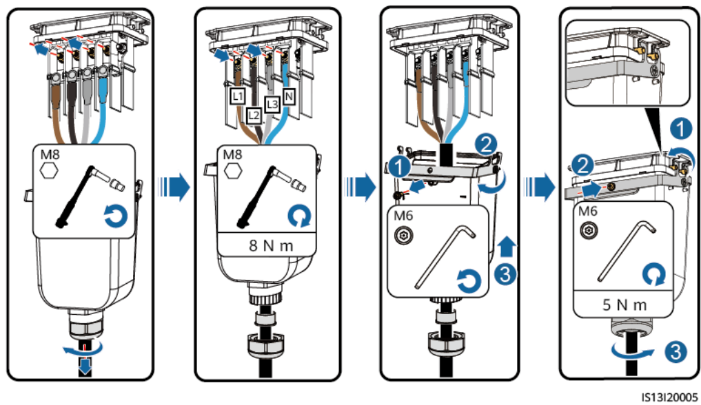
Figure 5-11 Câble à quatre conducteurs (L1, L2, L3 et N)
