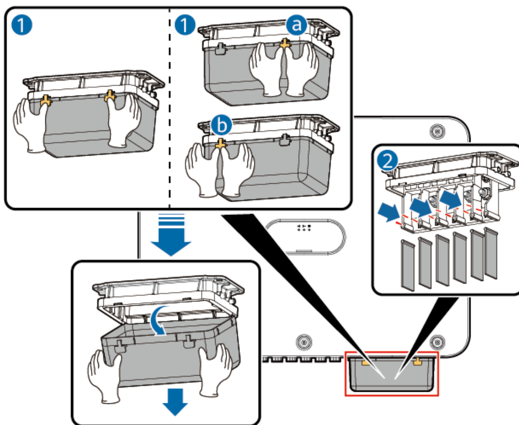
Figure 5-7 Retrait du boîtier de la borne CA
