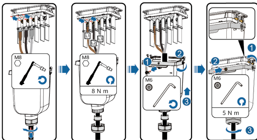
Figure 5-12 Câble à trois conducteurs (L1, L2 et L3)
