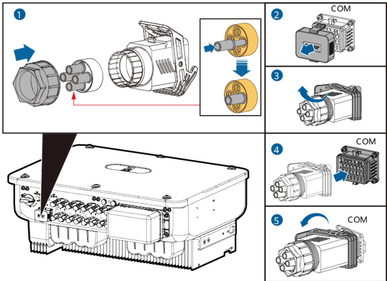
Figure 5-30 Connexion du connecteur du câble de signal
