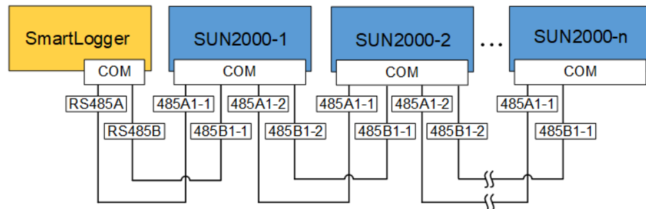
Figure 5-32 Mise en réseau du SmartLogger
