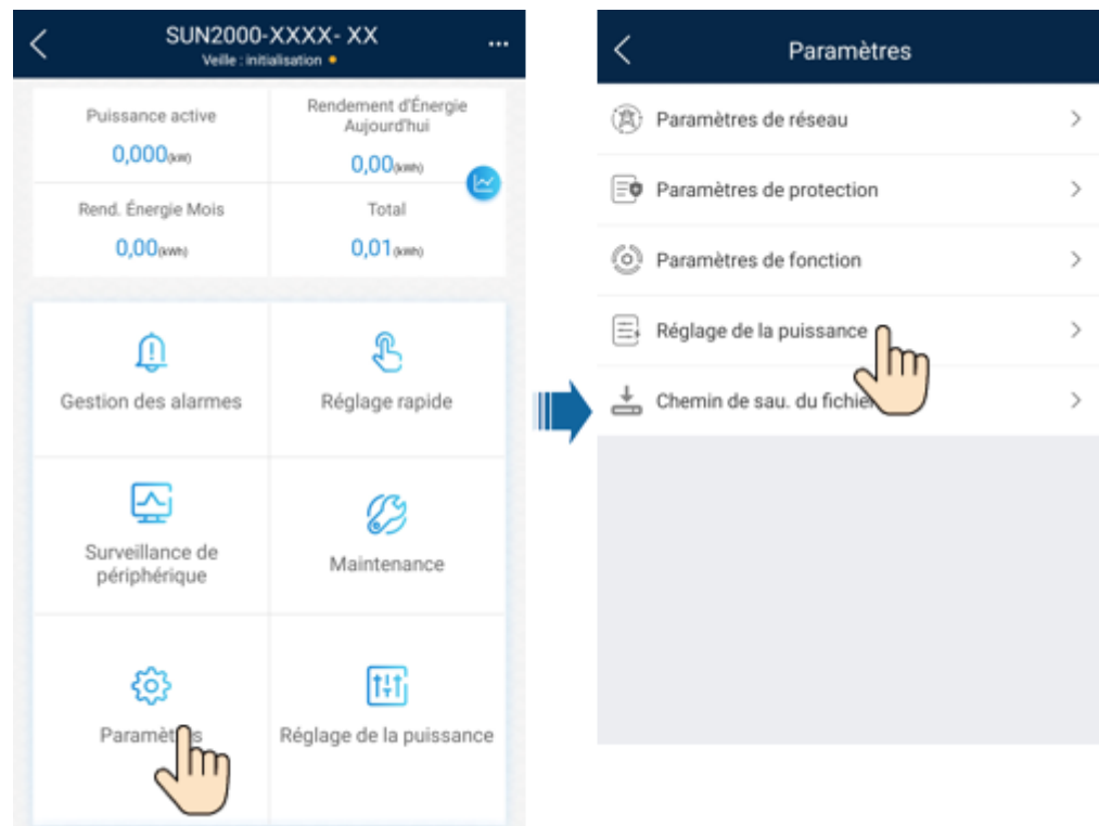
Figure 7-8 Contrôle de la puissance apparente
