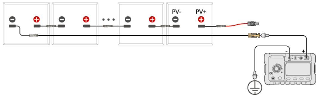
Figure 5-19 Mesure de la résistance d'isolation du PV- pour chaque chaîne PV
