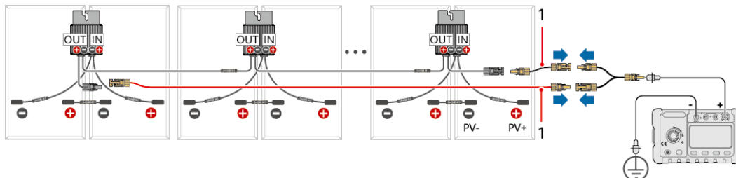
Figure 5-16 Mesure de la résistance d'isolation du câble d'extension
