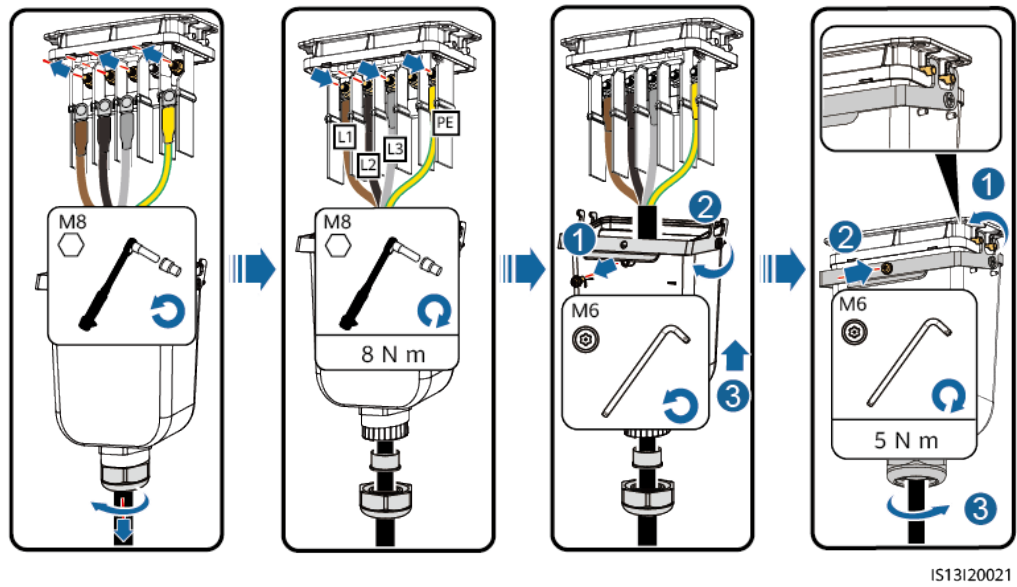
Figure 5-10 Câble à quatre conducteurs (L1, L2, L3 et PE)
