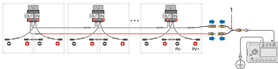
Figure 5-15 Mesure de la résistance d'isolation de chaque chaîne PV
