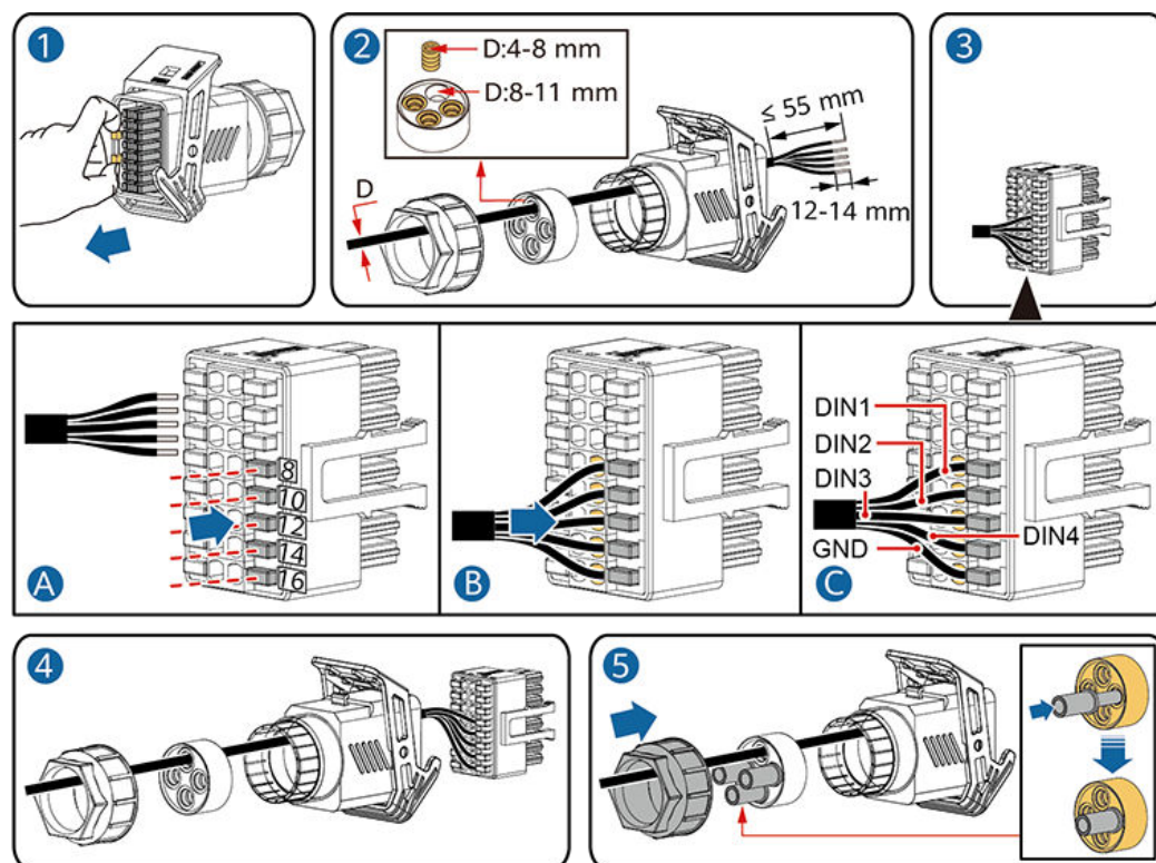
Figure 5-39 Connexion du câble
