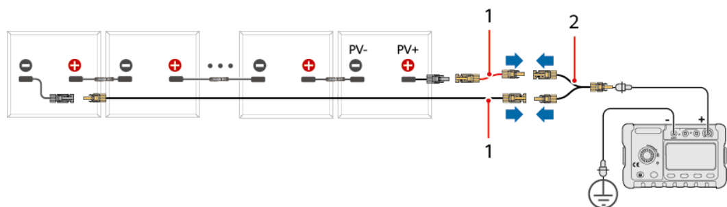
Figure 5-21 Mesure de la résistance d'isolation du câble d'extension
