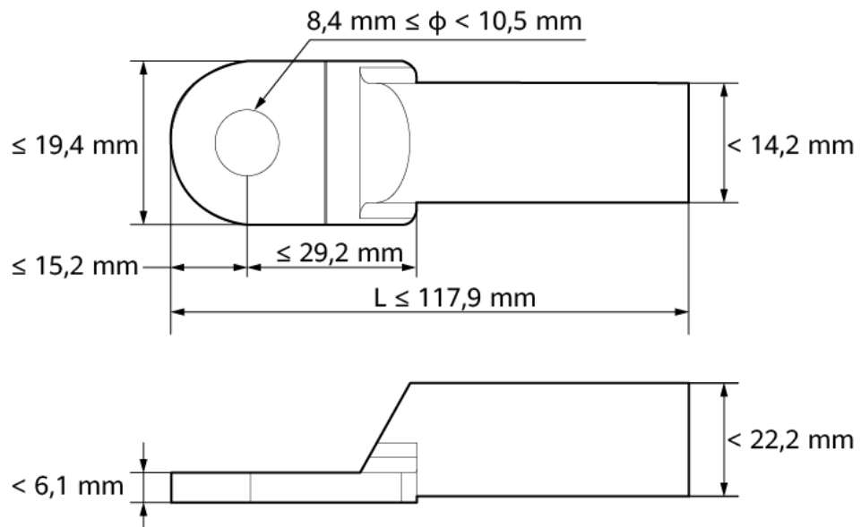
Figure 5-5 Caractéristiques de la borne OT/DT sertie
