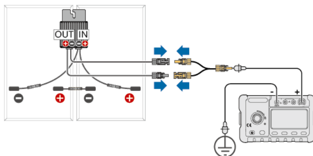
Figure 5-17 Mesure de la résistance d'isolation d'un module PV et de son optimiseur associé
