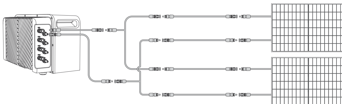
Connexion en parallèle
