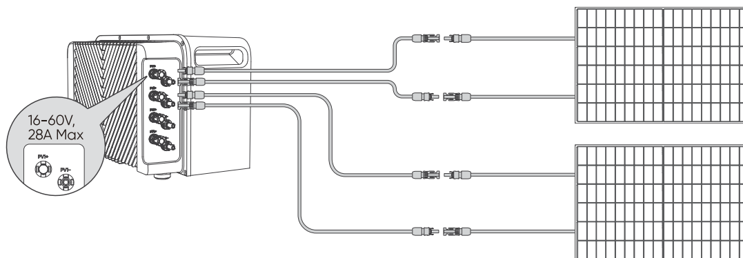
Connexion directe
