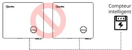
Un compteur ne peut pas être connecté à plusieurs onduleurs et différents transformateurs ne peuvent pas être connectés au même câble de ligne.
