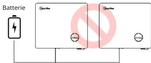
Une même batterie ne peut pas être connectée à plusieurs onduleurs.
