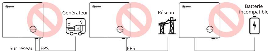
Ni le port EPS ni le port connecté au réseau ne doivent être directement connectés à un générateur.
