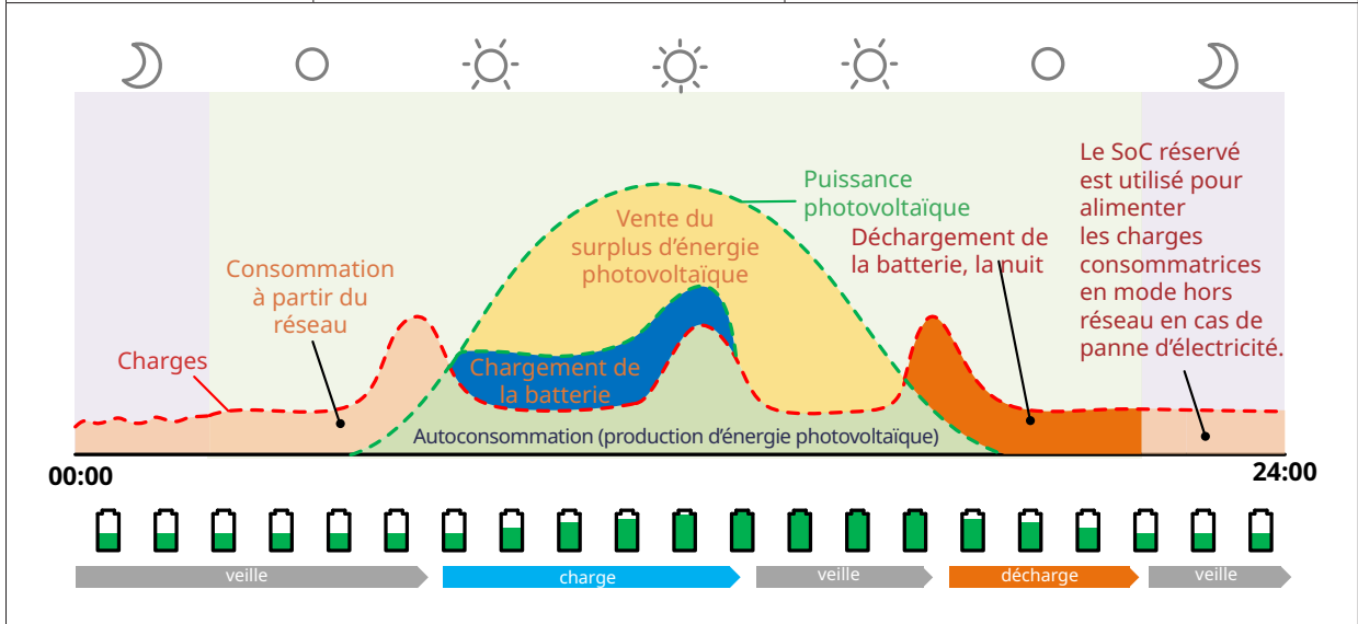
Évolution de la puissance en mode de secours
