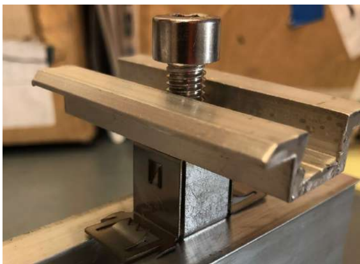
Bride JORISOLAR ST02 avec Terragrif PL
